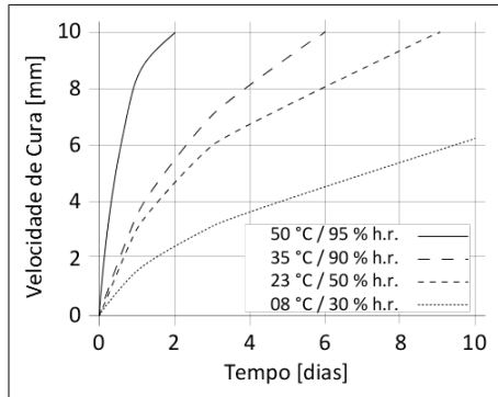
Diagrama 1: Velocidade de cura do Sikasil® IG-16
