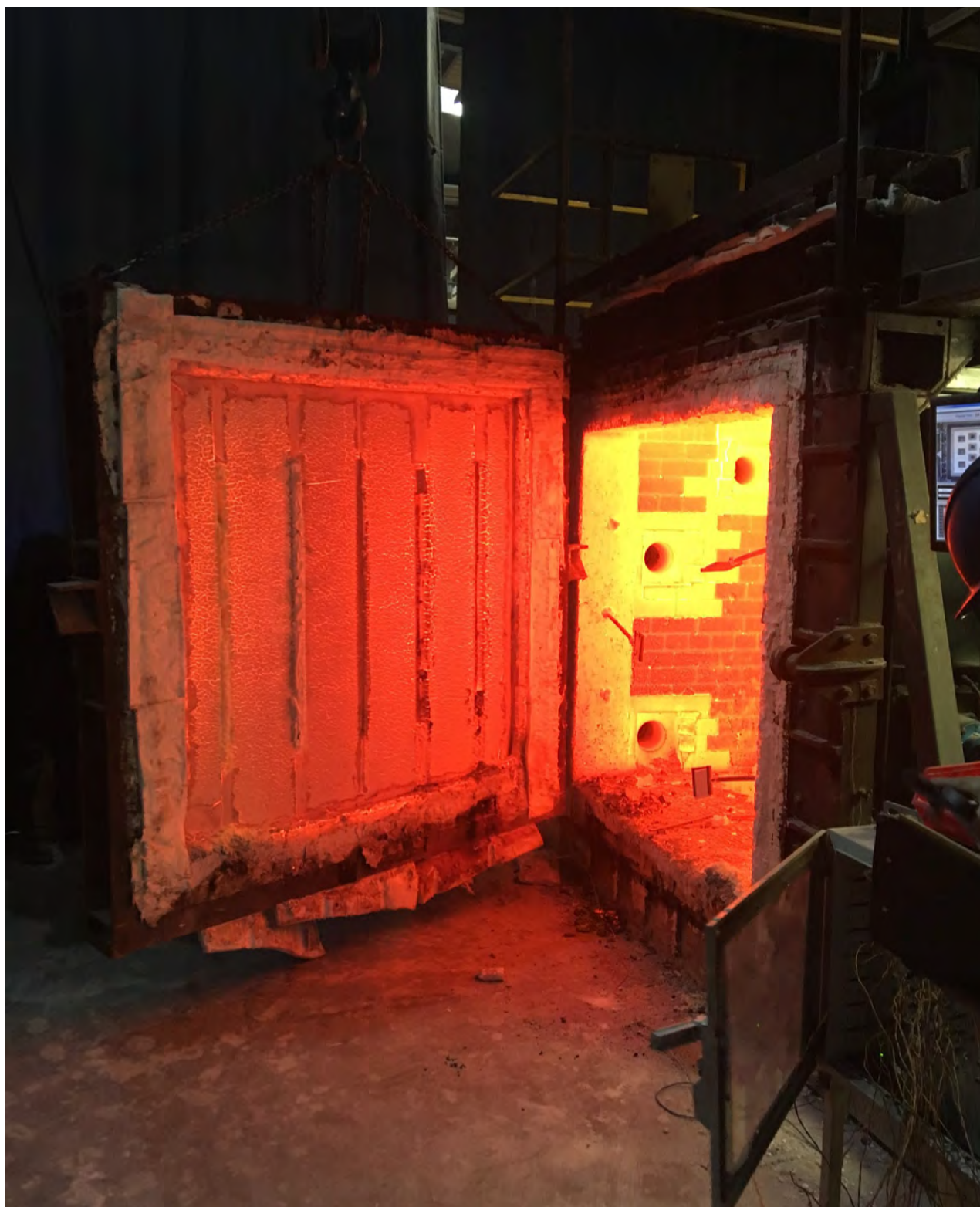
Fornalha com selagens lineares verticais após teste de resistência ao fogo segundo EN 1366-4
