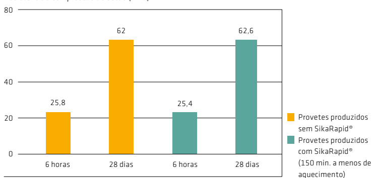
Resistência à compressão do betão (MPa)
