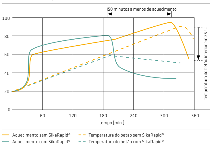
Desenvolvimento da temperatura do betão em °C
