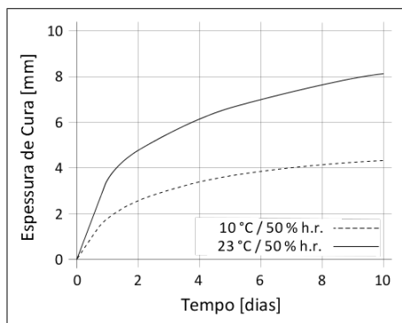
Diagrama 1: Velocidade de cura de Sikaflex®-552
