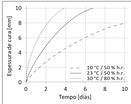
Diagrama 1: Velocidade de cura de SikaTack® Panel-50
