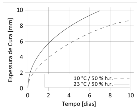
Diagrama 1: Velocidade de cura do SikaTack® MAX 30 (Purform®)
