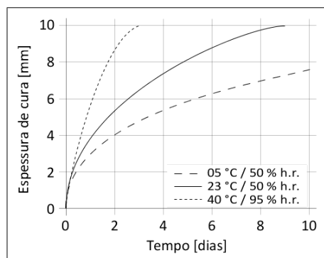
Diagrama 1: Velocidade de cura do Sikasil® WS-200.
